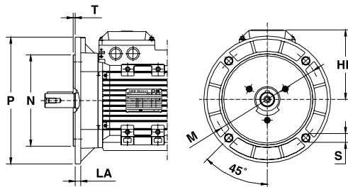
Flange-mounted motor, small flange; IM B14 (IM 3601)
