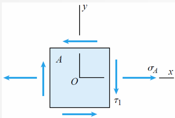
Estado de Tensão no ponto A
